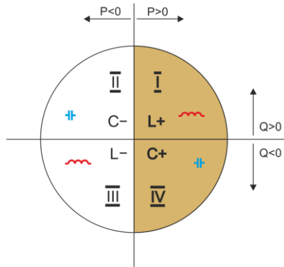
Fig. 18. La división del flujo de potencia y energía de cuatro cuadrantes.
