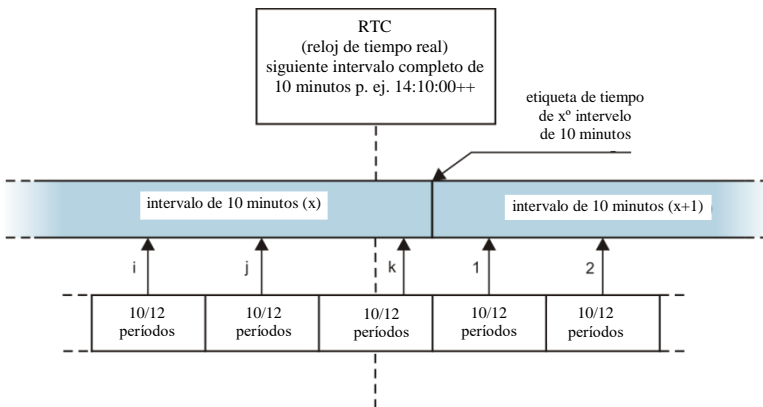
Fig. 23. Determinación de períodos del cálculo de media más largos (o iguales) a 10 segundos (por ejemplo para 10 minutos)
