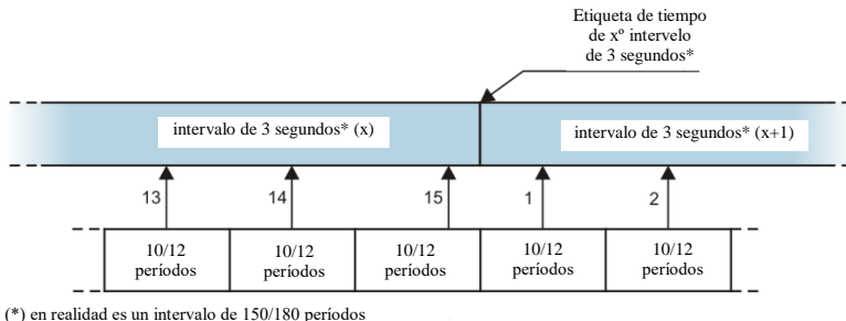
Fig. 24. Determinación de intervalos de cálculo de media más cortos que 10 segundos (por ejemplo para el cálculo de promediación de 3 segundos)
