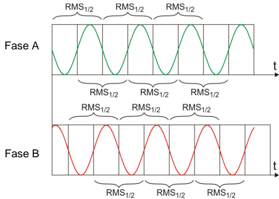
Fig. 21. Determinación del valor U_{RMS(1/2)}
