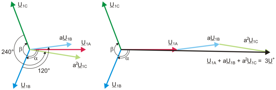
Fig. 19. Ejemplo de determinación de componente de secuencia positiva.
