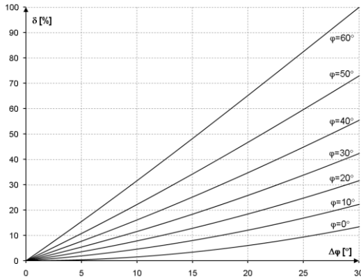
Fig. 25. La incertidumbre adicional resultante del error de fase, dependiendo del ángulo de desplazamiento de fase.
