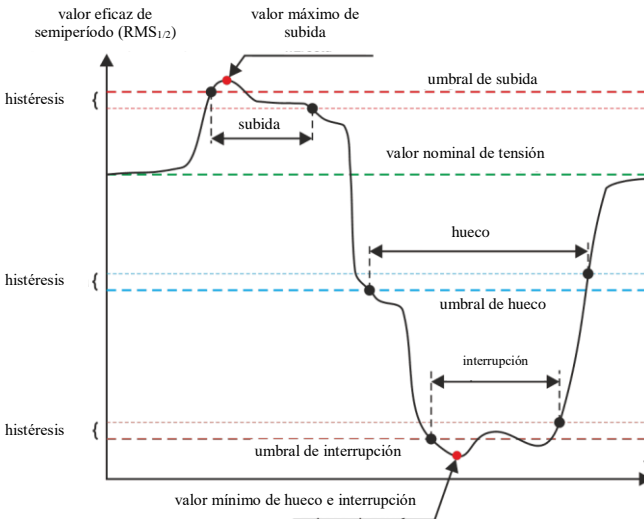
Fig. 20. Subidas, huecos e interrupciones de tensión.
