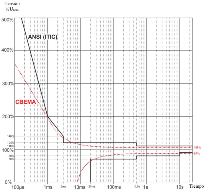
Fig. 22. Curvas de tolerancia de tensión de alimentación ANSI (ITIC) y CBEMA.
